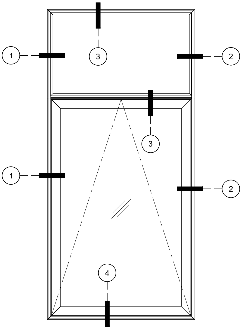
Tampak Luar
